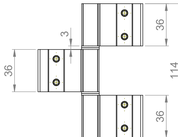
DIMENSÕES (ESCALA 1:2)
