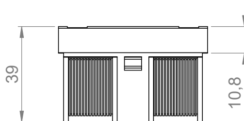
DIMENSÕES (SEM ESCALA)
