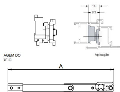
ABERTURA DE 90° (PARA LIMPEZA E REGULAGEM DO FREIO)
