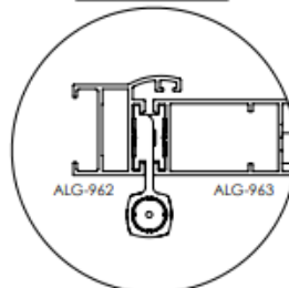
DETALHE B ESCALA 1 : 2
