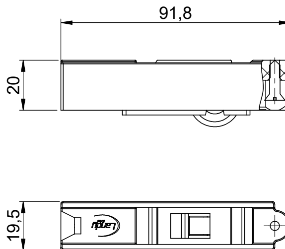
DIMENSÕES (ESCALA 1:1.5)
