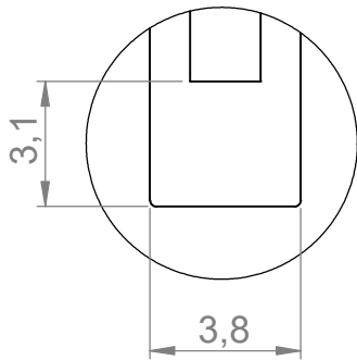
DETALHE C
