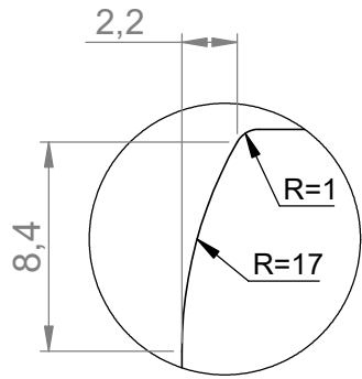
DETALHE A
