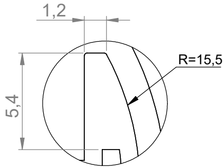
DETALHE B
