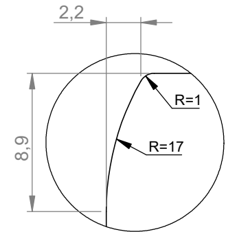
DETALHE A
