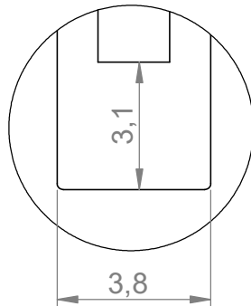
DETALHE C
