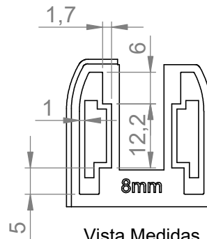
Vista Medidas do Encaixe
