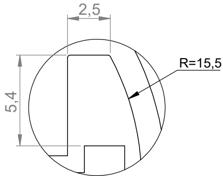
DETALHE B
