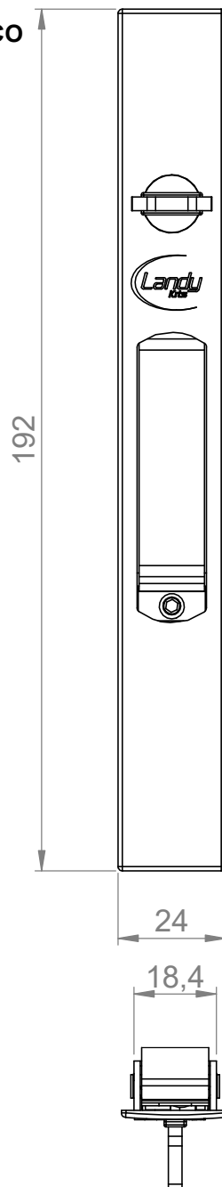
USINAGEM ESQUADRIA (SEM ESCALA)
