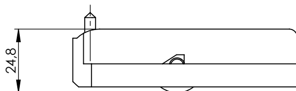
REGULAGEM MÍNIMA
