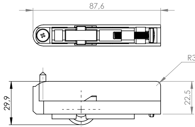
REGULAGEM MÁXIMA
