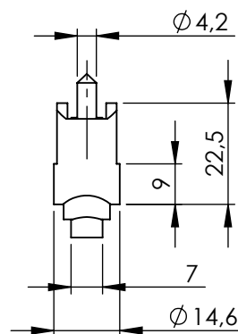
REGULAGEM MÁXIMA
