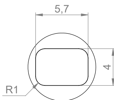
DETALHE D
