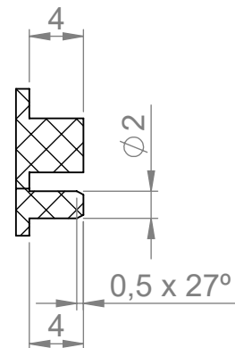
SEÇÃO A-A
