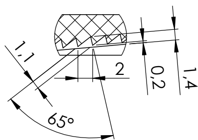
DETALHE B ESCALA 2 : 1
