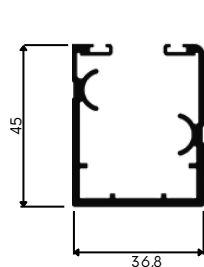
TRILHO INFERIOR
