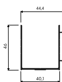
PERFIL "U" DE REGULAGEM
