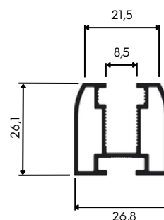
PERFIL CAPA
