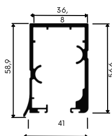
TRILHO SUPERIOR
