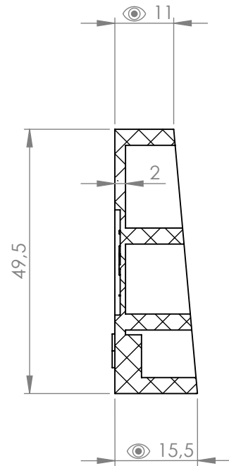
SEÇÃO A-A
