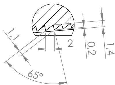
DETALHE B ESCALA_2 : 1
